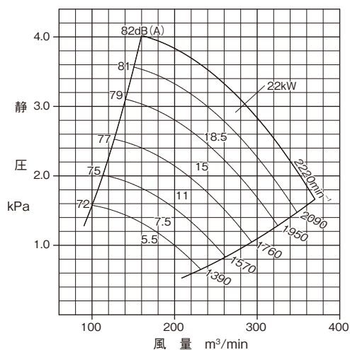
CTFII-No.4½
