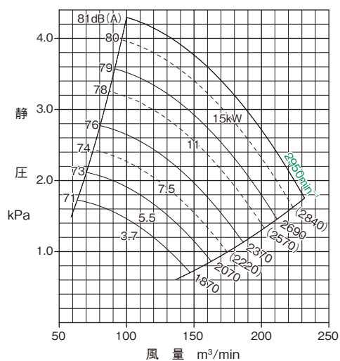
CTFII-No.4½
