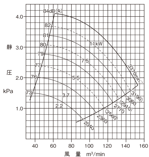
CTFII-No.4
