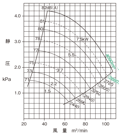
CTFII-No.3½
