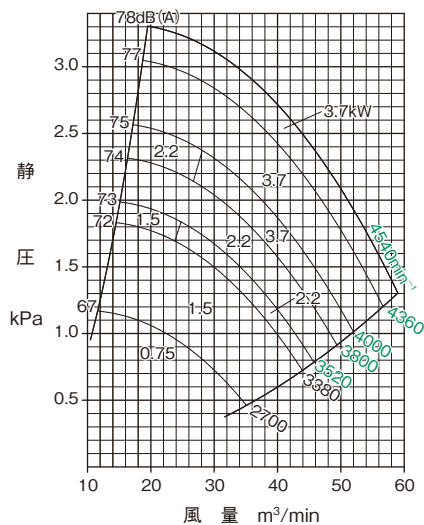
CTFII-No.3
