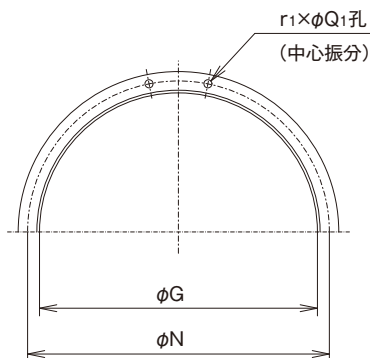
吸込相フランジ
